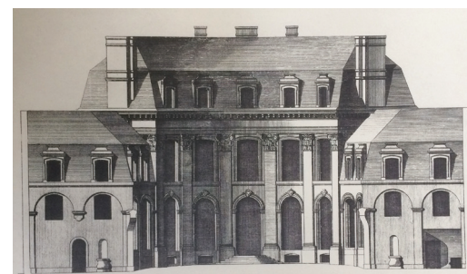
Élévation de la façade sur cour de l'hôtel de Gournay, tirée de L'architecture française de Jean Mariette, 1727, republié par Louis Hauteceœur en 1929 © Alice Cronier
